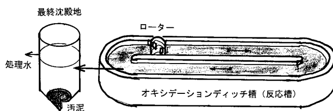
オキシデーションディッチ構造説明図
